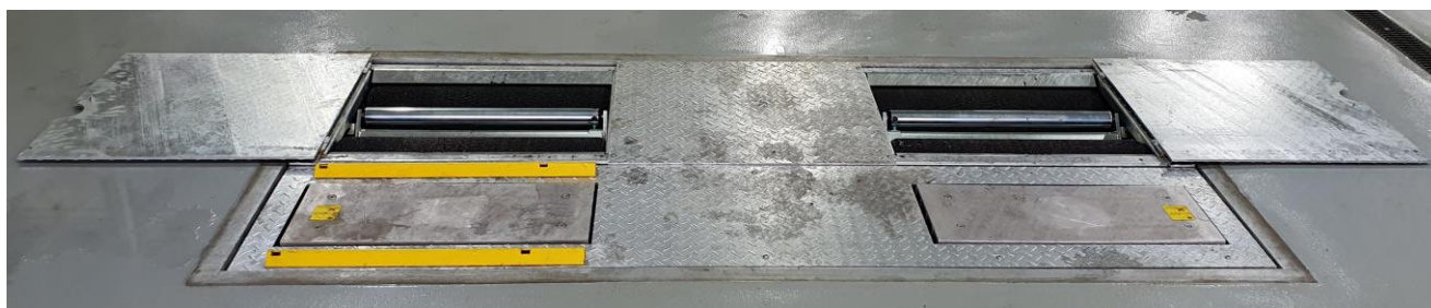
BEISSBARTH VAS 6360-PC - testovací linka podvozku - brzda 4x4 + zkušebna tlumičů
