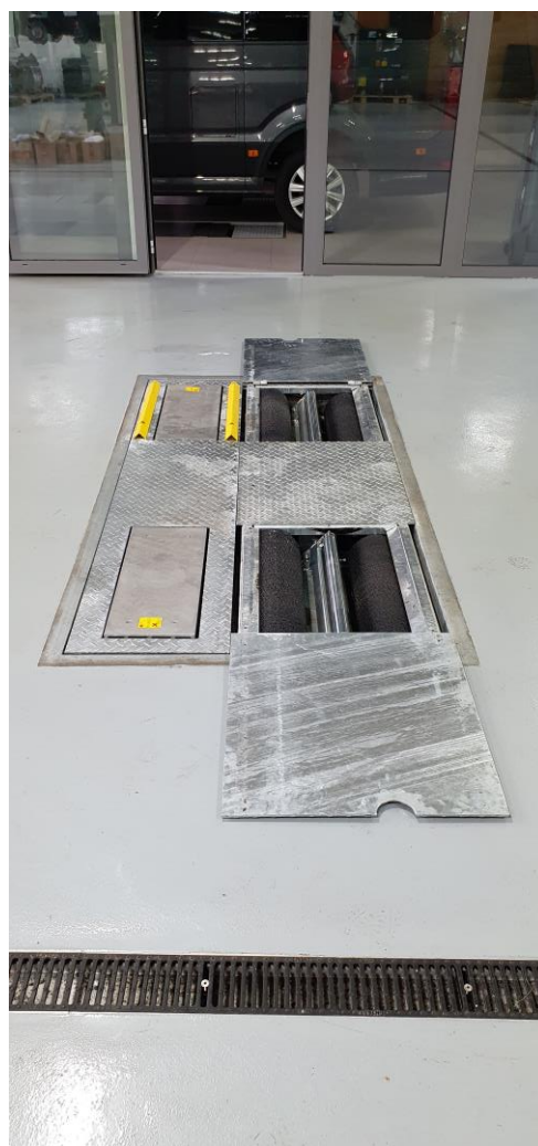
BEISSBARTH VAS 6360-PC - testovací linka podvozku - brzda 4x4 + zkušebna tlumičů
